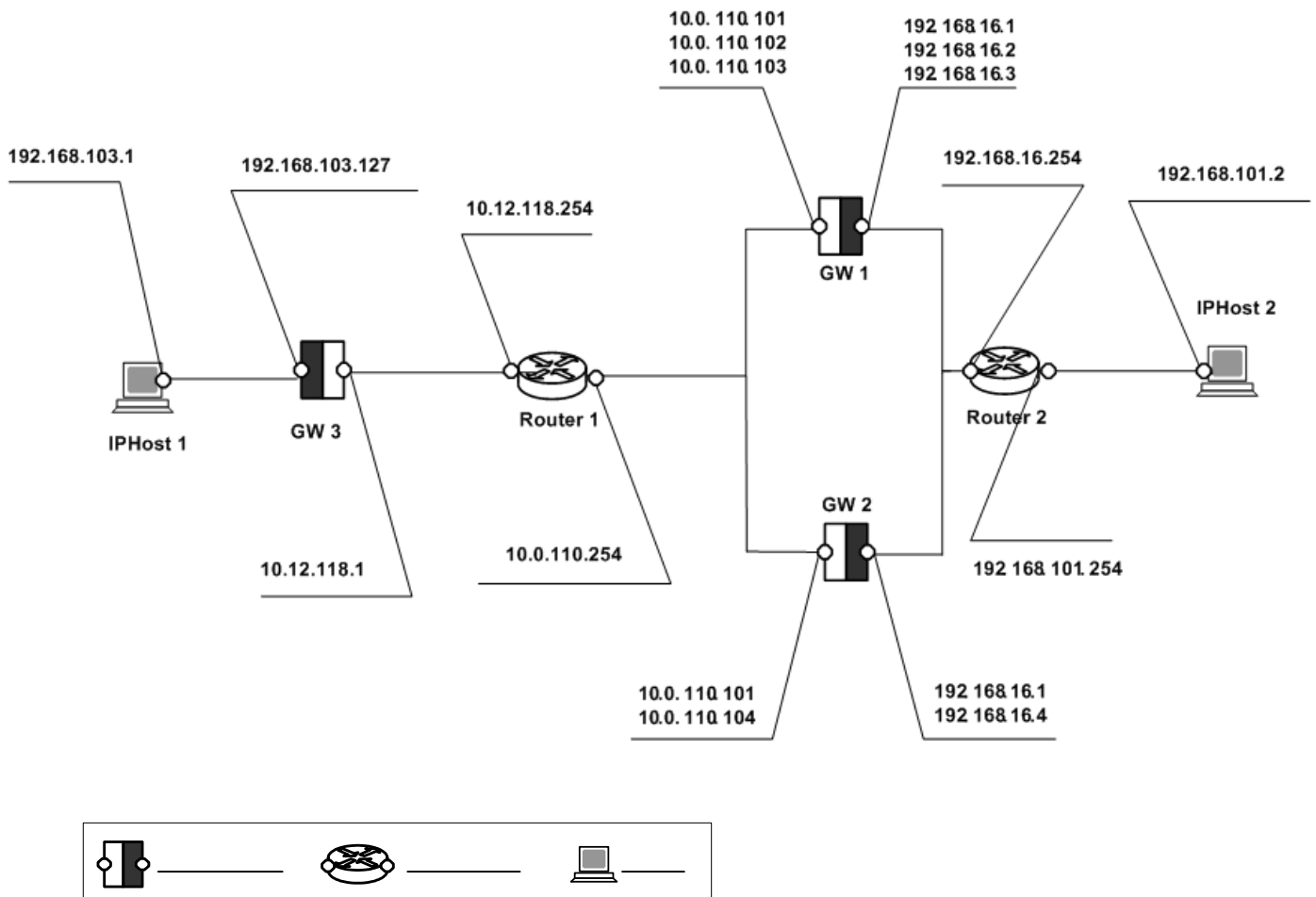
Рис. 2 Схема стенда
