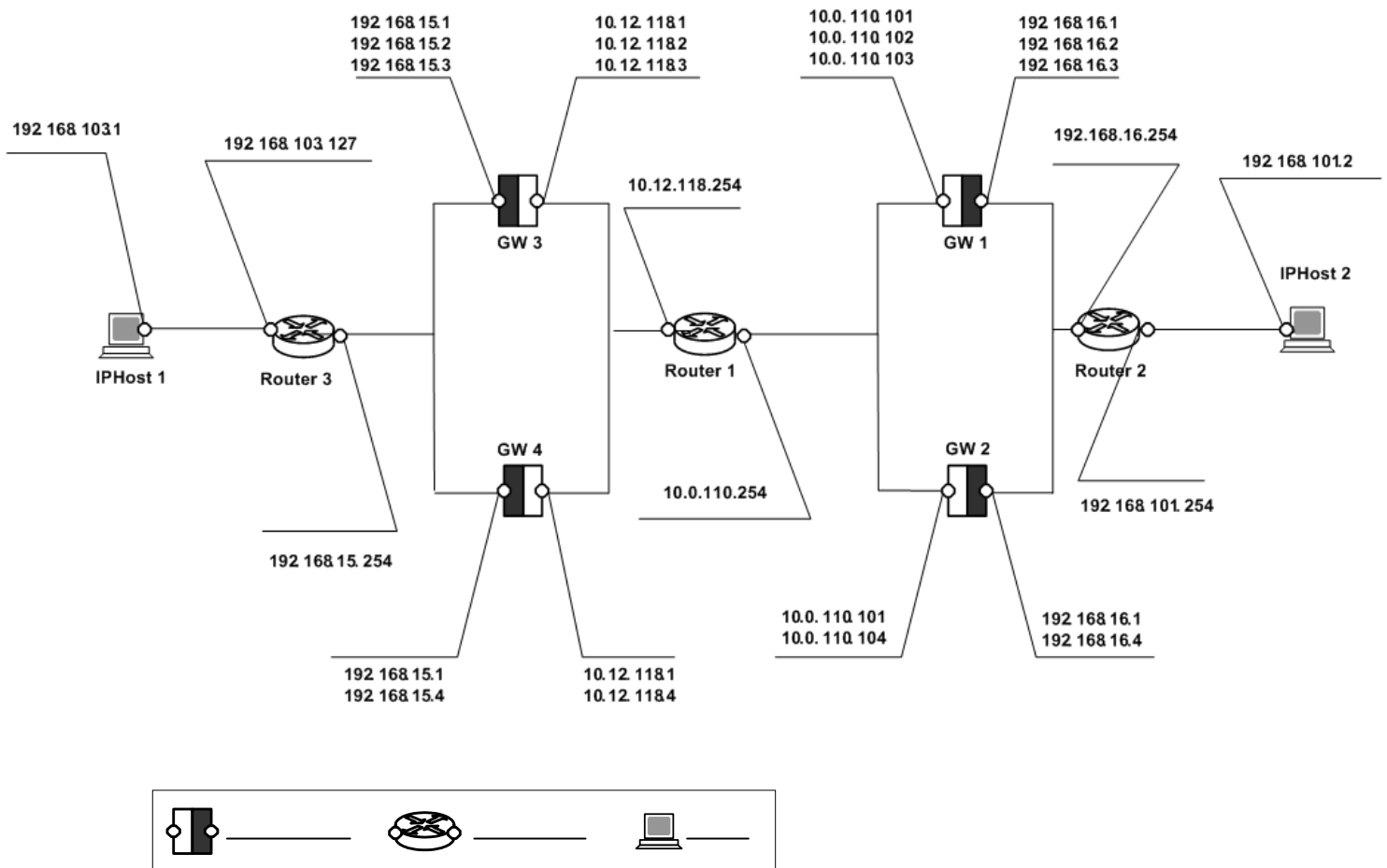
Рис. 2 Схема стенда
